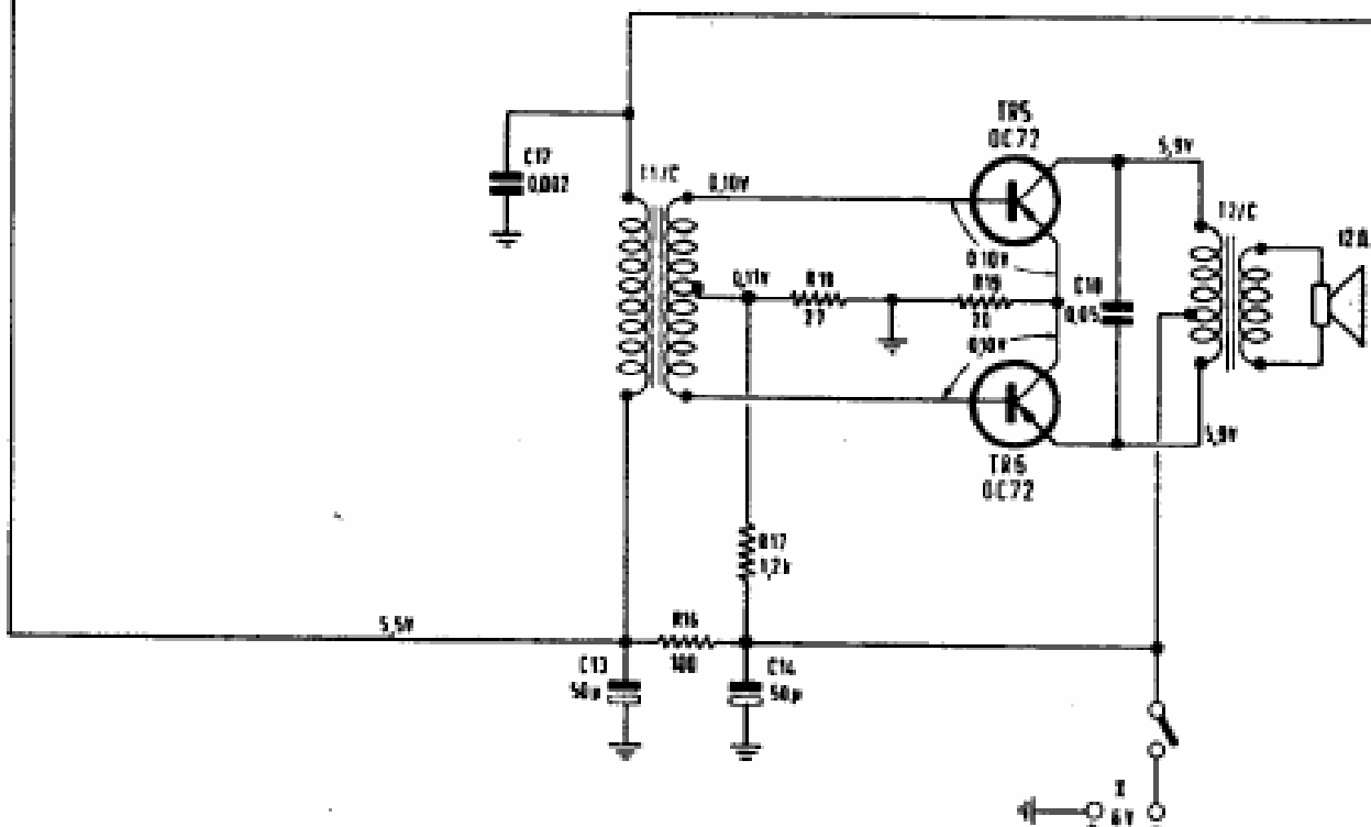
Schema elettrico del radio ricevitore a transistori ATLANTIC - Mod. T 267 - 269
